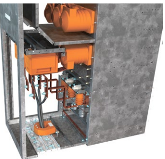
КРУ-СВЭЛ двустороннего обслуживания
