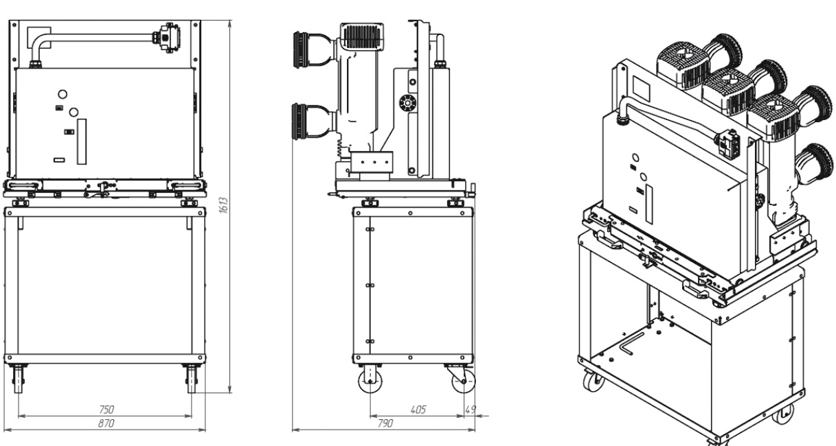
Максимальная масса инвентарной тележки с установленным вакуумным выключателем номиналом от 630 А до 1250 А составляет 170 кг
