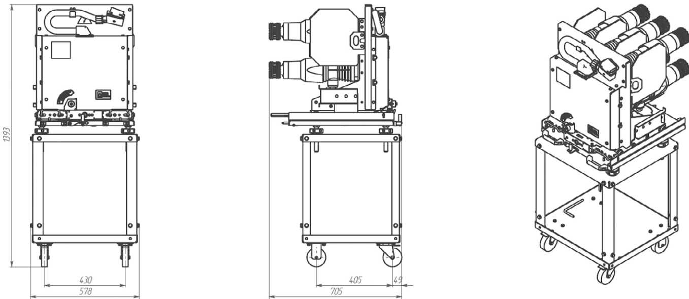
Максимальная масса инвентарной тележки с установленным вакуумным выключателем номиналом от 630 А до 1250 А составляет 170 кг
