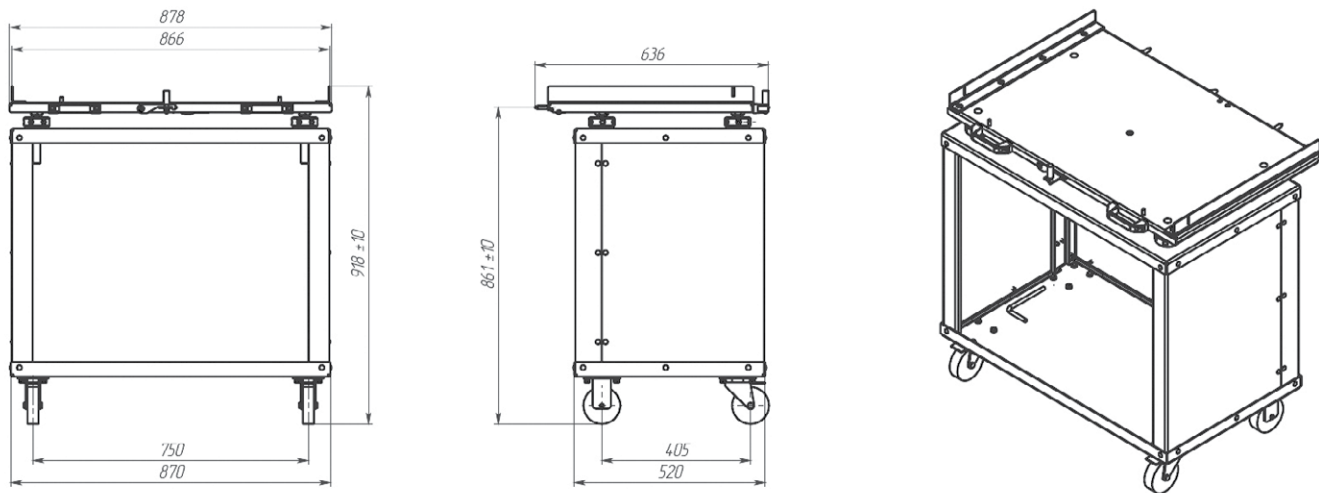
Масса инвентарной тележки для вакуумных выключателей номиналом от 630 А до 1250 А составляет 40 кг
