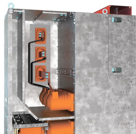
КРУ-СВЭЛ двустороннего обслуживания
