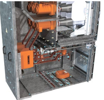
КРУ-СВЭЛ одностороннего обслуживания
