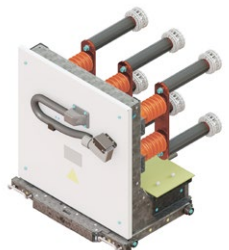
КВЭ с секционным разъединителем
